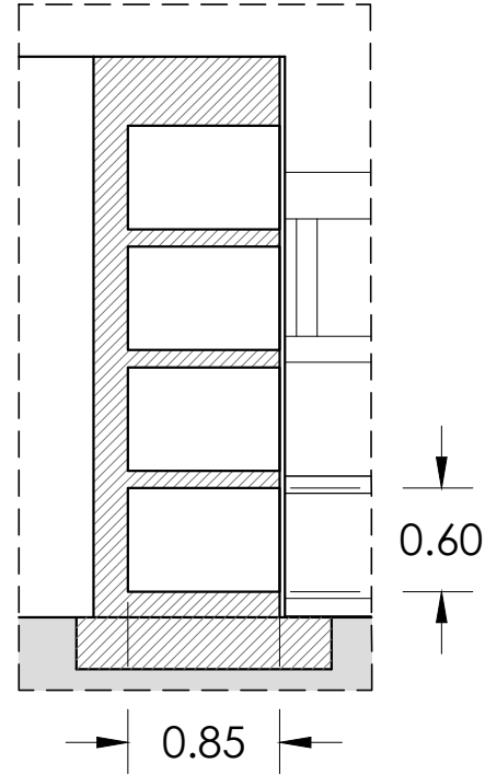
BLOCCO TIPO - SEZIONE
