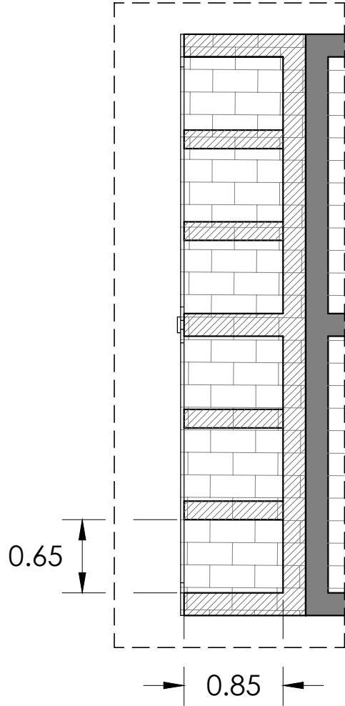
BLOCCO TIPO - PIANTA
